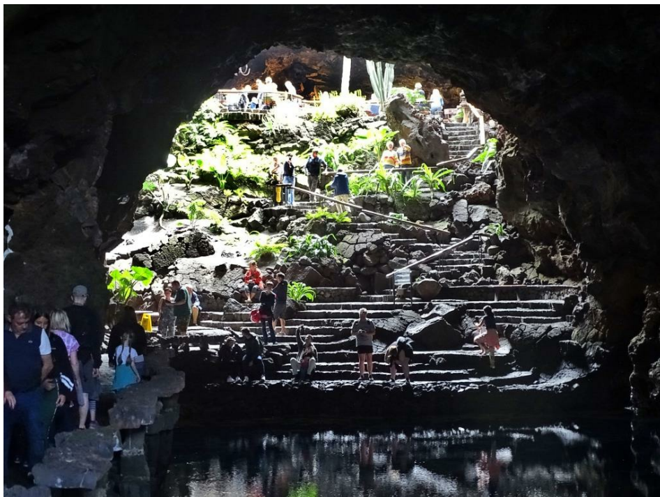
Lavatunnel mit Höhlensee
