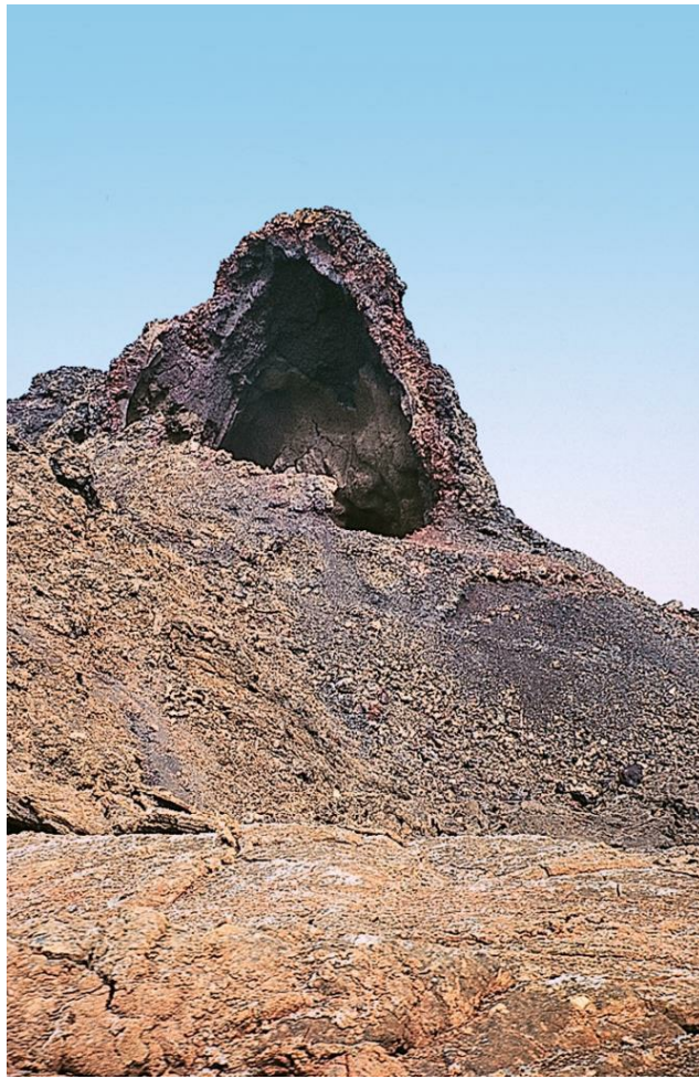
Hornito in den Feuerbergen
